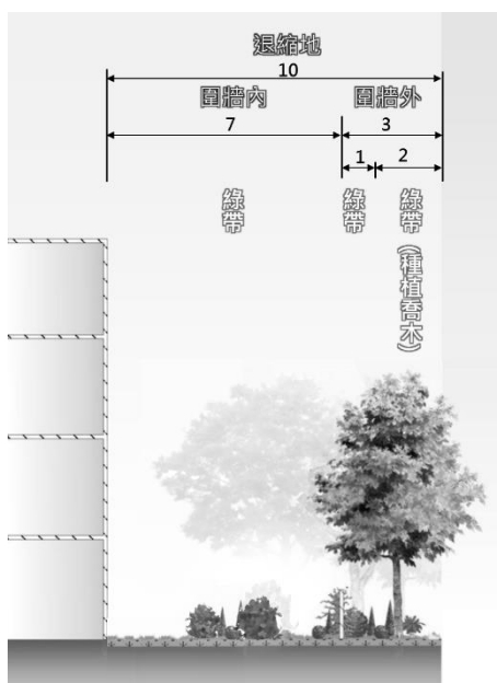
B. 臨 20 公尺寬以上道路之退縮地使用管制示意圖
